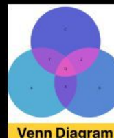
Venn Diagram
